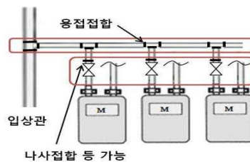
그림 2.5.8.5.4(1) “건축물 내의 집합 계량기 배관 접합부의 경우”
